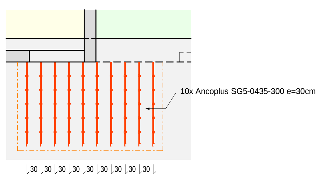
Detail B 1 : 50 Schubbewehrung
