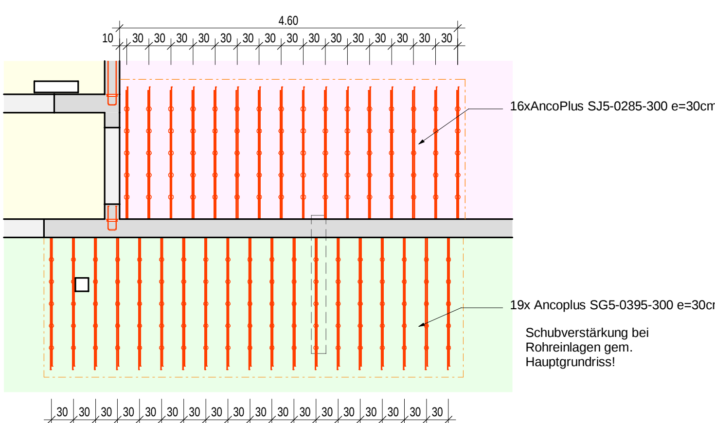
Detail A 1 : 50 Schubbewehrung
