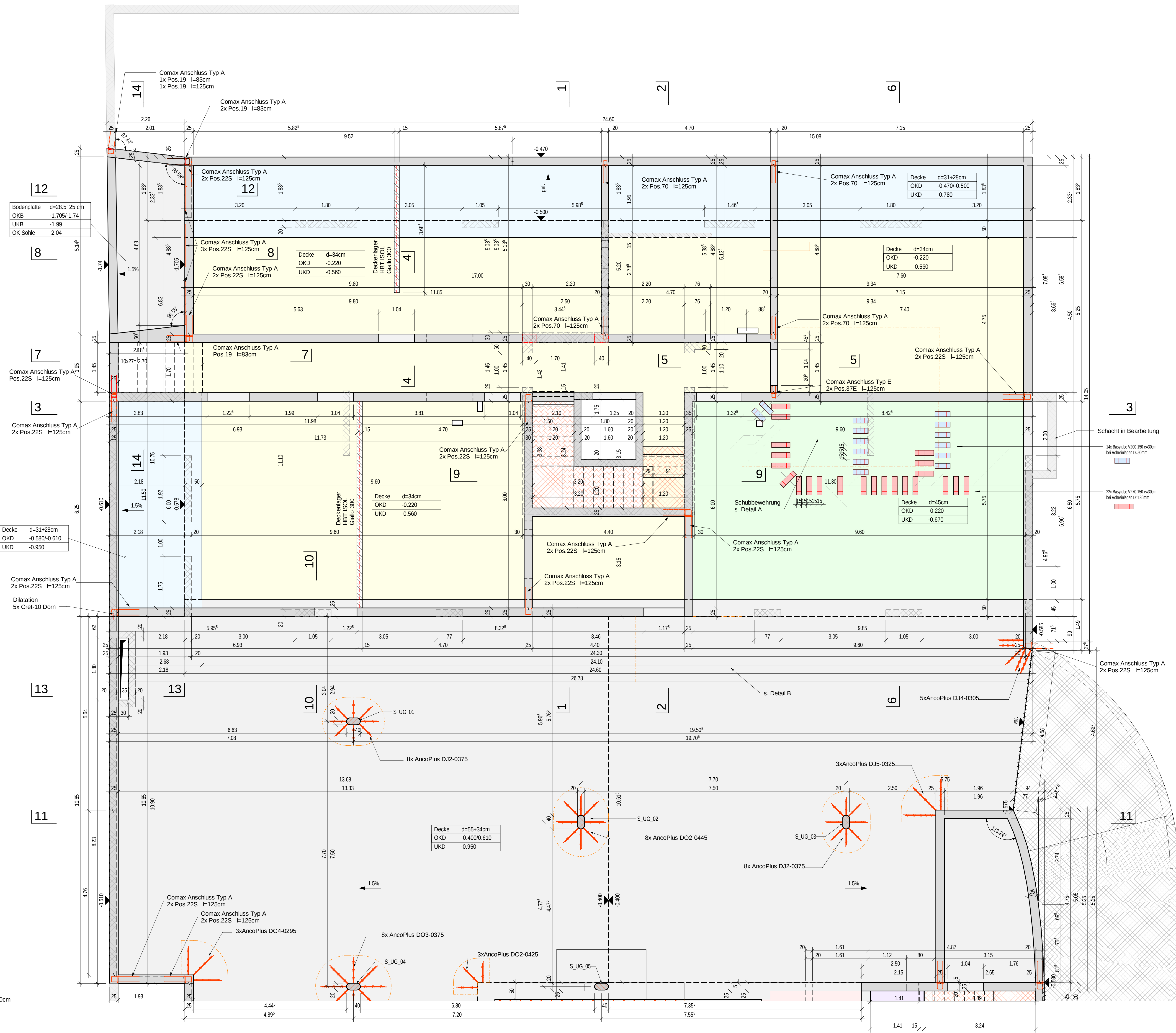
Grundriss Decke Bushaltestelle 1 : 50
