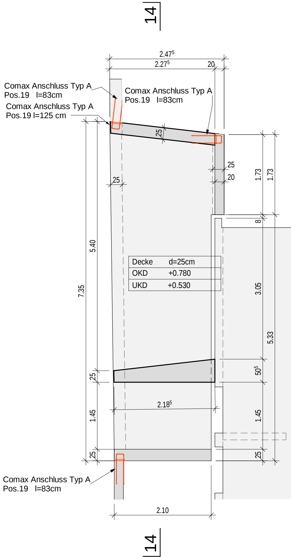
Grundriss Decke Bushaltestelle 1 : 50
