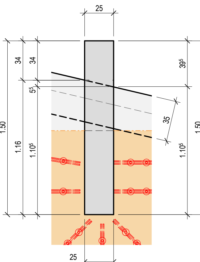
Teilgrundriss Ortbeton Pfeiler 1 : 20
