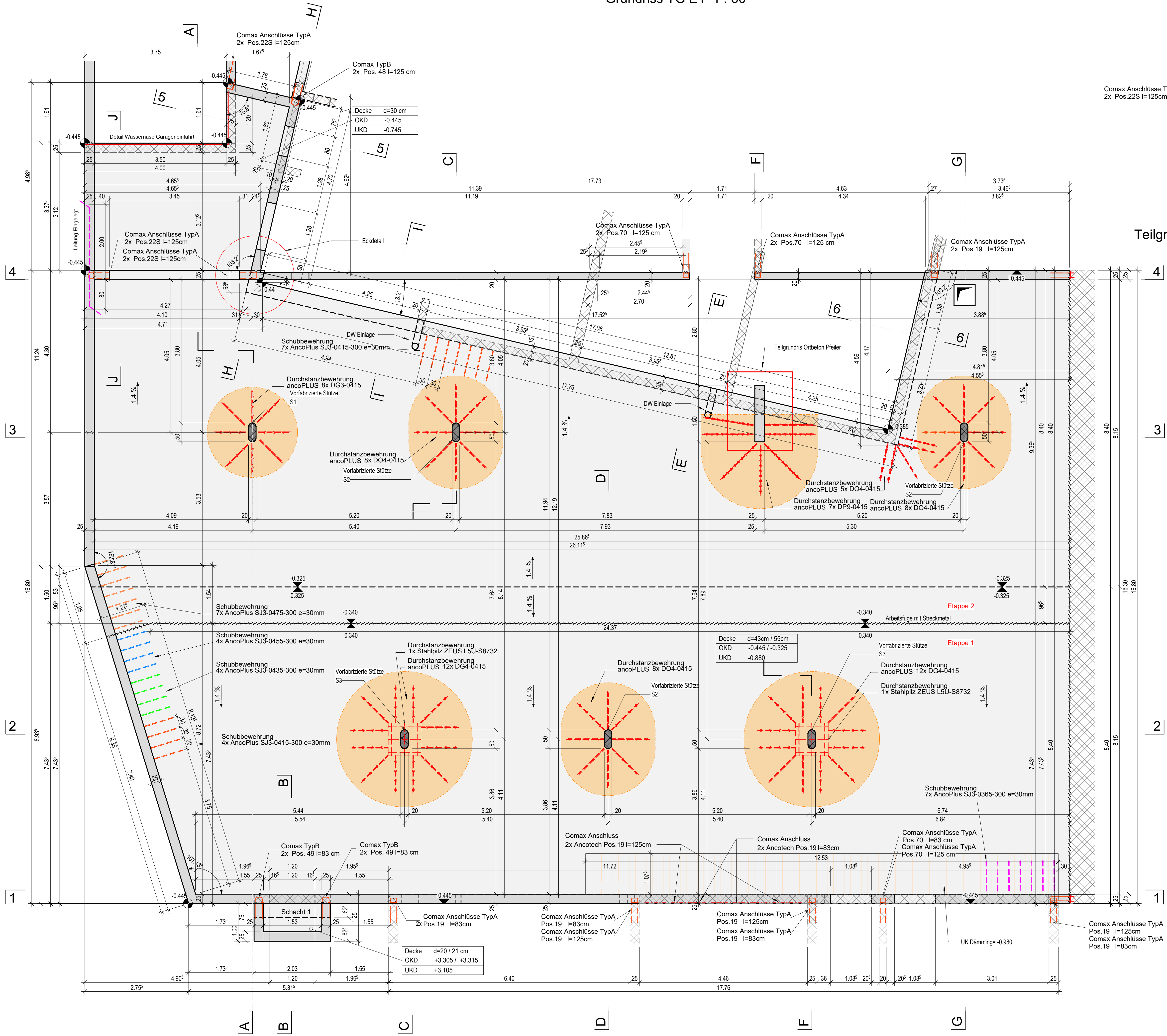
Grundriss TG E1 1 : 50
