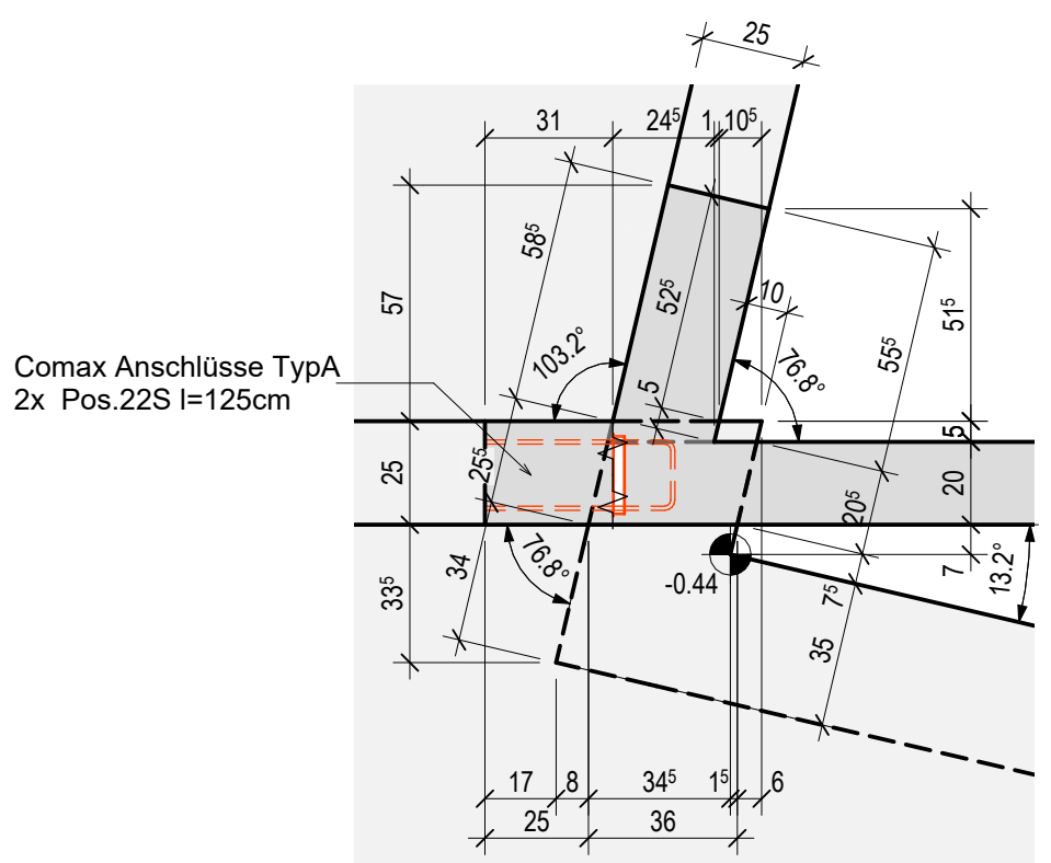
Grundriss Eckdetail 1 : 20
